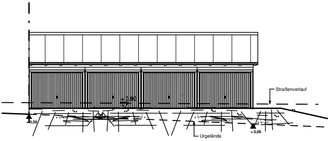
Ansicht von Westen
