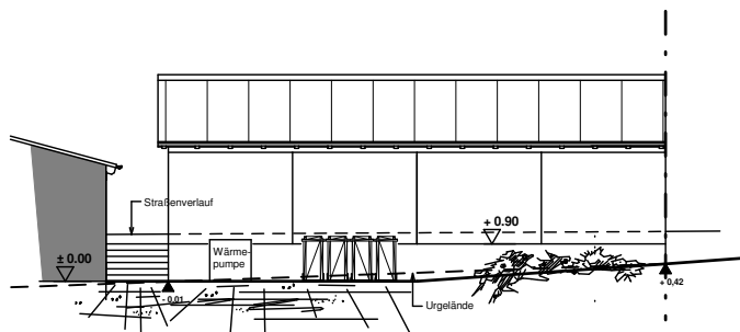
Ansicht von Osten
